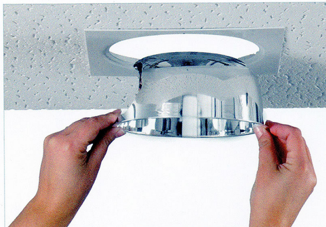
3 Retirar difusor (siempre que sea posible).
