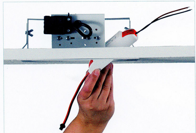
4: Colocar alimentador en falso techo y conectar a red
